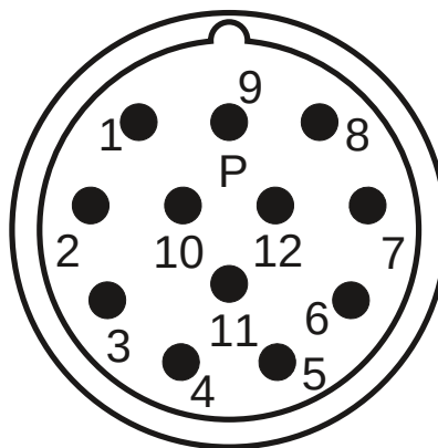
Konektor 2 (293)
