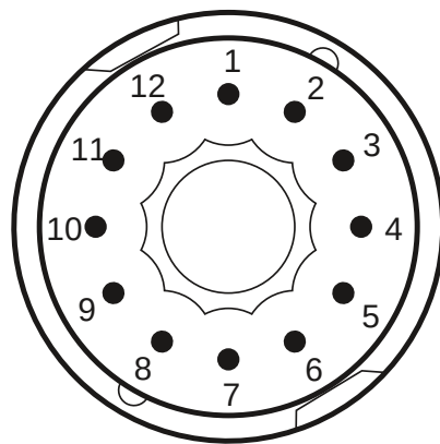
Connector 2 (208)
